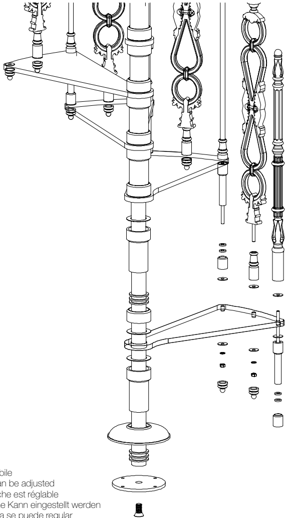
(A) Alzata gradino in cm. - Step height in cm - Stufenhöhe in cm. - Contremarche en cm. - Contrahuella del escalón en cm
